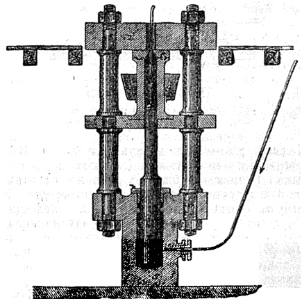
Фиг. 3. Прессованіе свинцовыхъ трубъ.
