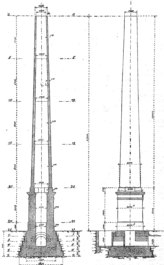
Круглая заводская труба.
