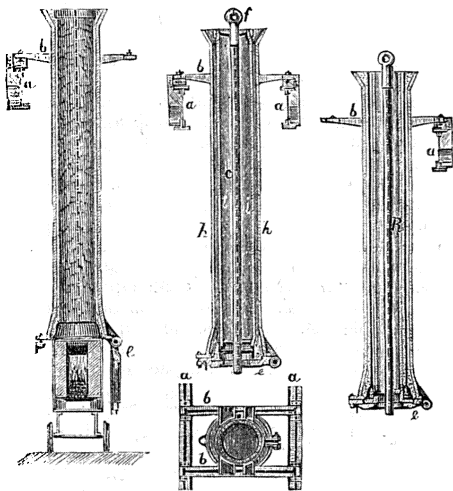
Фиг. 1. Формовка чугунныхъ трубъ.
