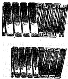
Фиг. 6. Гибкія металлическія трубы.
