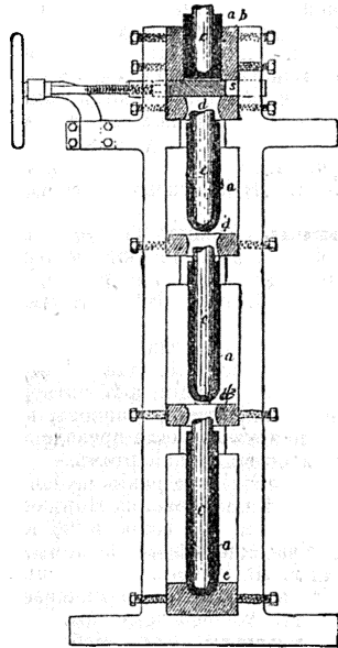
Фиг. 2. Изготовленіе трубъ безъ шва по способу Эргарта.
