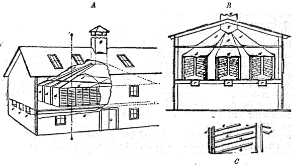
Фиг. 2 Патентованная сушильня для рыбы системы Витмана. А — общій видъ. В — разрѣзъ по линіи аа С — деталь расположенія полокъ для рыбы (а) и трубу (б), по которымъ циркулируетъ вода.
