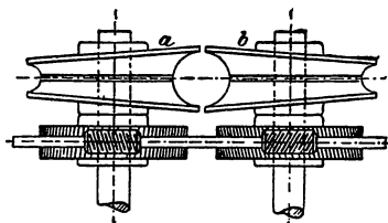
Фиг. 5. Валки для изготовленія рифленыхъ коническихъ трубъ.
